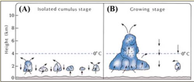
ಚಿತ್ರ 19. (A) ಬೇರೆ ಬೇರೆಯಾಗಿರುವ ಮೋಡದ ಚಿಕ್ಕ ತುಂಡುಗಳು. (B) ಚಿಕ್ಕ ಚಿಕ್ಕ ಮೋಡಗಳು ಒಟ್ಟು ಸೇರುವಾಗ, ದೊಡ್ಡ ಮೋಡದೊಳಗಿನ ಮೇಲೇರುವ ಒತ್ತಡದ ಗಾಳಿ ಹೆಚ್ಚಾಗುತ್ತದೆ. ಇದರಿಂದಾಗಿ ಮೋಡವು ಮೇಲ್ಬೃಷ್ಟವಾಗಿ ಪೇರಿಸಲ್ಪಡುತ್ತದೆ. ನೀರಿನ ಬಿಂದುಗಳನ್ನು ಚುಕ್ಕಿಗಳ ಮೂಲಕ ತೋರಿಸಲಾಗಿದೆ. [The Atmosphere, Anthes and others, p. 269.]
