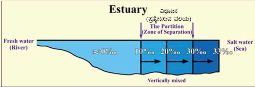
ಚಿತ್ರ 14. ನದೀಮುಖದಲ್ಲಿ ಲವಣಾಂಶವನ್ನು (ಪ್ರತಿ ಸಹಸ್ರ % ಭಾಗಗಳಲ್ಲಿ) ತೋರಿಸುವ ರೇಖಾಂಶ ಚಿತ್ರ. ಶುದ್ಧನೀರು ಮತ್ತು ಉಪ್ಪುನೀರಿನ ಮಧ್ಯೆಯಿರುವ ವಿಭಾಜಕ (ಪ್ರತ್ಯೇಕಿಸುವ ವಲಯ)ವನ್ನು ಇಲ್ಲಿ ಕಾಣಬಹುದಾಗಿದೆ. [Introductory Oceanography, Thurman, p. 301, with a slight enhancement.]
